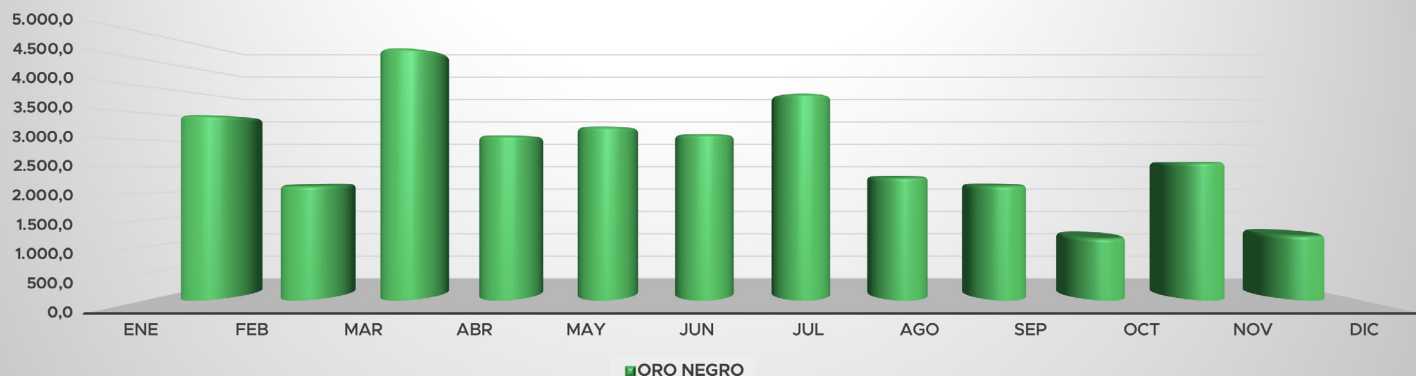
ELABORACIÓN DE GASOLINA BLANCA EN REFINERÍA ORO NEGRO - GESTIÓN 2021 (Expresado en m3/mes)
