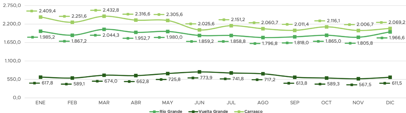
PRODUCCIÓN DE PLANTAS DE PROCESOS DE G.N. CON FACILIDADES DE EXTRACCIÓN DE GLP - GESTIÓN 2021 (Expresado en Toneladas Métricas)
