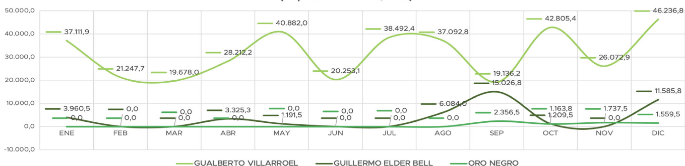
ELABORACIÓN DE GASOLINA BASE 81 EN REFINERÍAS - GESTIÓN 2021 (Expresado en m3/mes)
