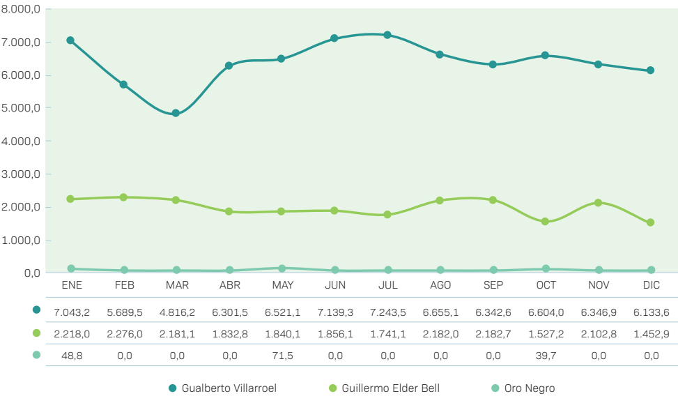
ELABORACIÓN DE GLP EN REFINERÍAS - GESTIÓN 2024 (Expresado en m³/mes)
