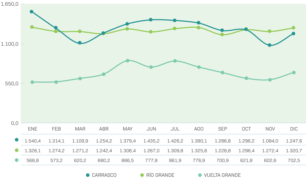
PLANTAS DE PROCESOS DE G.N. CON FACILIDADES DE EXTRACCIÓN DE GLP - GESTIÓN 2024 (Expresado en Toneladas Métricas)
