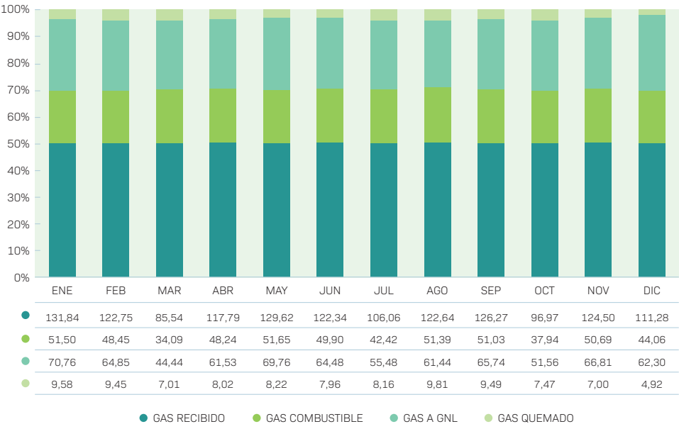
PLANTA DE GAS NATURAL LICUADO (PGNL) ALIMENTACIÓN DE GAS - PLANTA SEPARACIÓN DE LÍQUIDOS (MMPCD) - GESTIÓN 2024 (Participación Porcentual)
