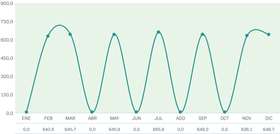
ELABORACIÓN DE GASOLINA DE AVIACIÓN EN REFINERÍA GUALBERTO VILLARROEL - GESTIÓN 2024 (Expresado en m³/mes)
