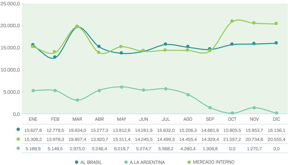
TRANSPORTE DE GAS POR GASODUCTOS - GESTIÓN 2024 (Expresado en Millones de Pies Cúbicos)
