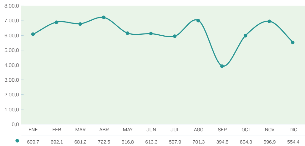
ELABORACIÓN DE BUTANO EN REFINERÍA GUILLERMO ELDER BELL - GESTIÓN 2024 (Expresado en BPD)
