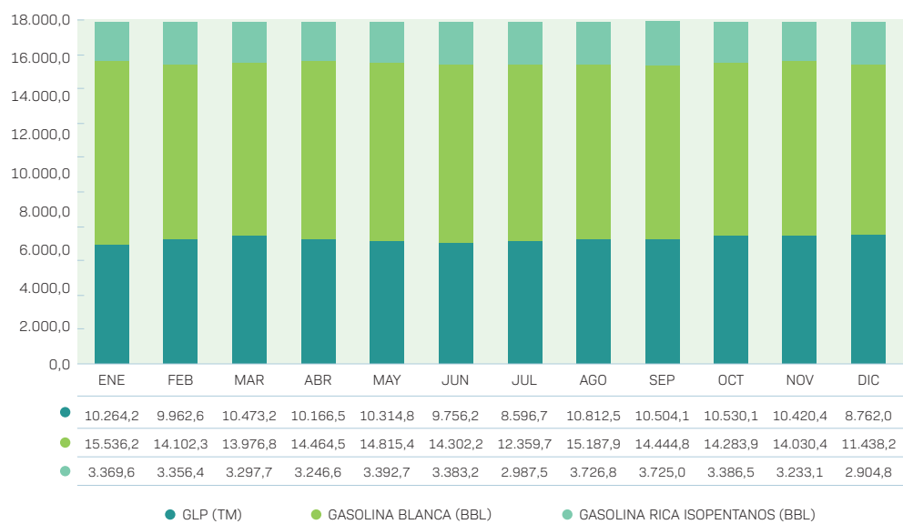
PRODUCCIÓN EN PLANTA SEPARADORA DE LÍQUIDOS RÍO GRANDE - GESTIÓN 2024 (Expresado en TM/BBL)
