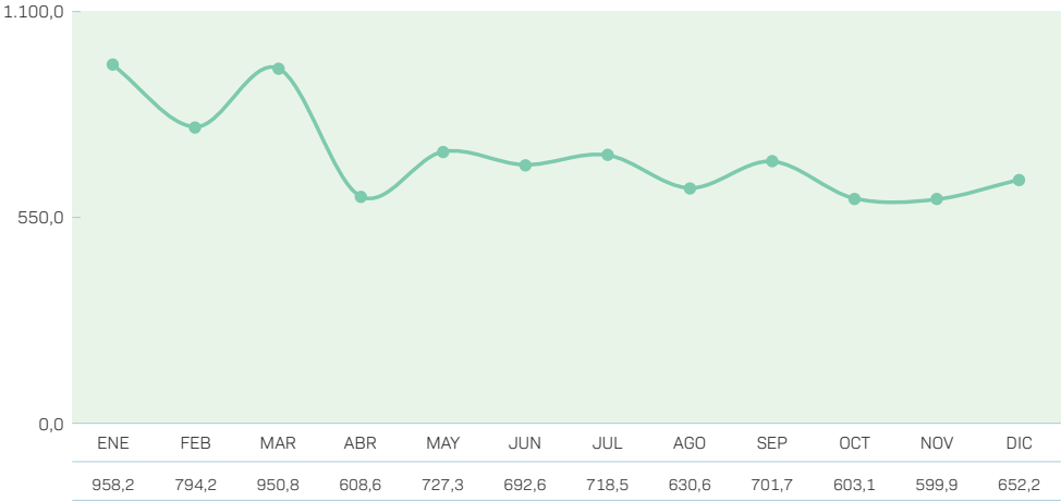
Cuadro No. 20 ELABORACIÓN DE NAFTA LIVIANA EN REFINERÍA ORO NEGRO - GESTIÓN 2024 (Expresado en m³/mes)
