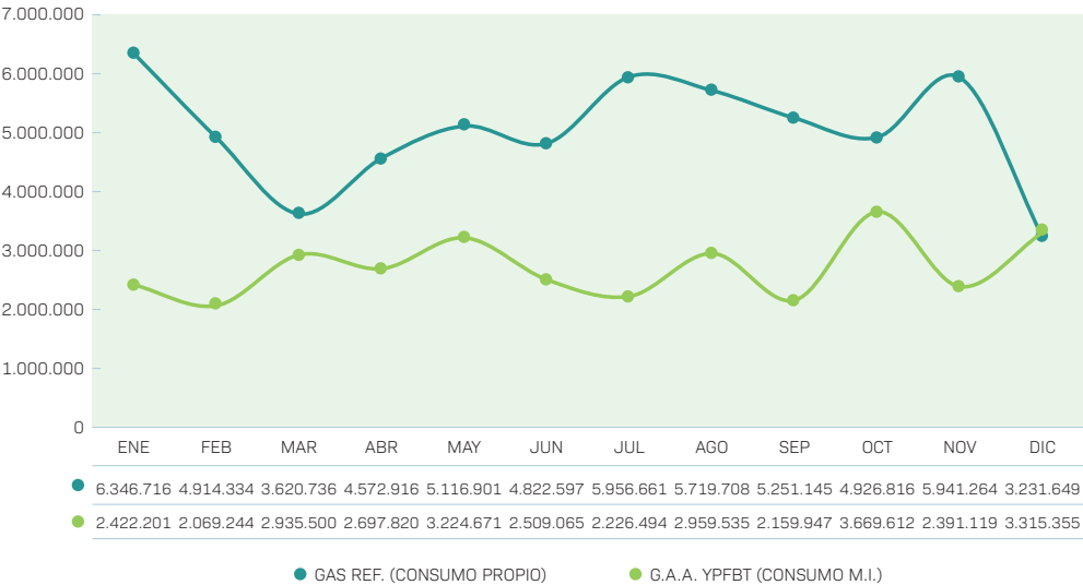
CONSUMO DE GAS EN REFINERÍA GUALBERTO VILLARROEL - GESTIÓN 2024 (Expresado en m³/mes)
