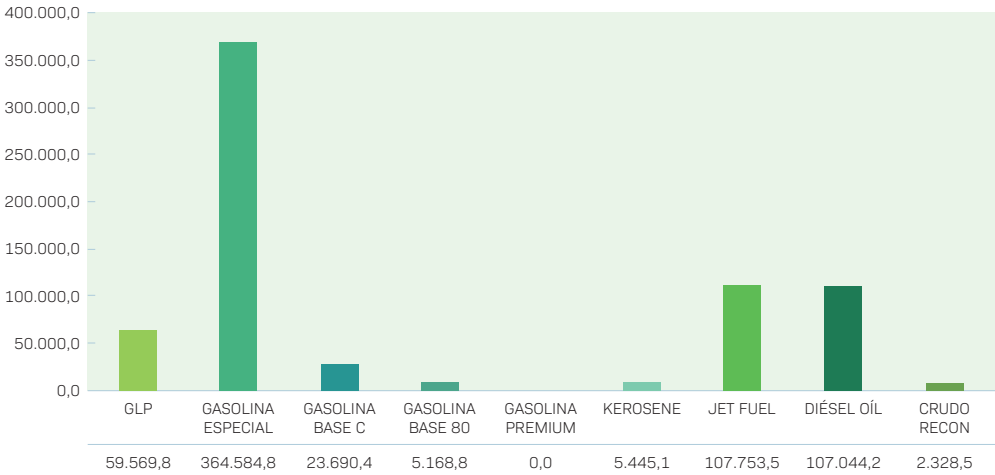
PRODUCCIÓN EN REFINERÍA GUILLERMO ELDER BELL - GESTIÓN 2024 (Expresado en Metros Cúbicos)
