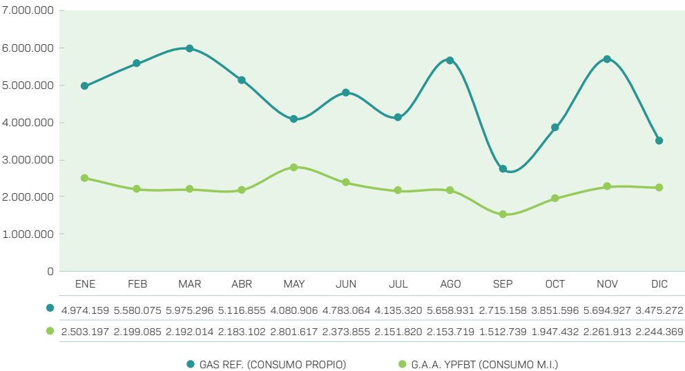
CONSUMO DE GAS EN REFINERÍA GUILLERMO ELDER BELL - GESTIÓN 2024 (Expresado en m³/mes)
