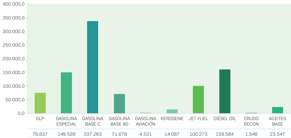
PRODUCCIÓN EN REFINERÍA GUALBERTO VILLARROEL - GESTIÓN 2024 (Expresado en Metros Cúbicos)
