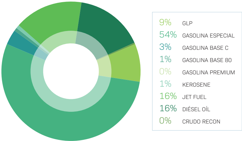
PRODUCCIÓN EN REFINERÍA GUILLERMO ELDER BELL - GESTIÓN 2024 (Participación Porcentual)
