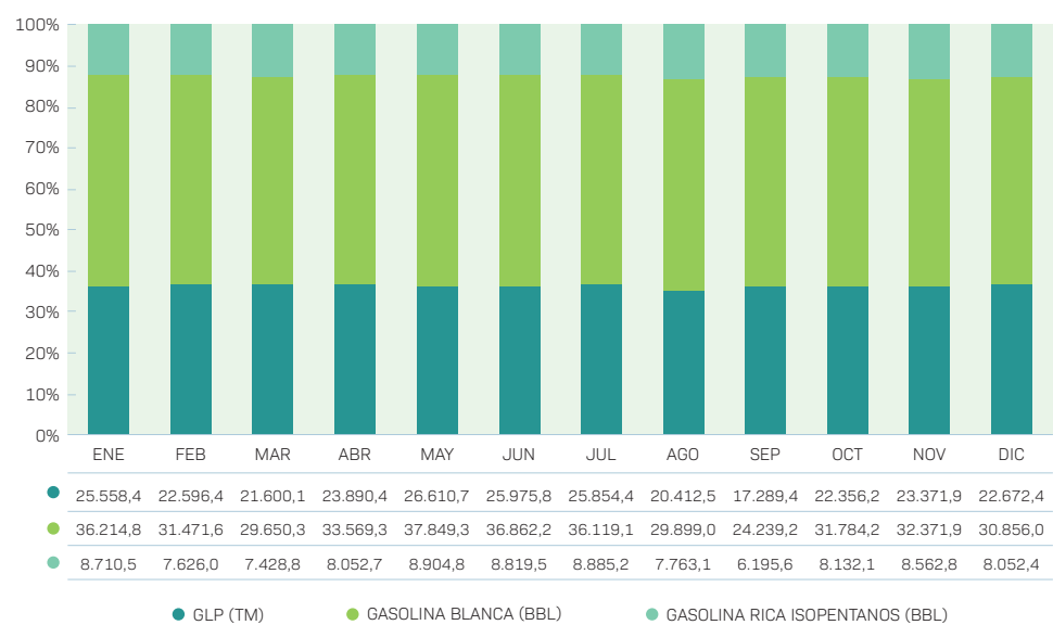
PRODUCCIÓN EN PLANTA SEPARADORA DE LÍQUIDOS CARLOS VILLEGAS - GESTIÓN 2024 (Expresado en TM/BBL)
