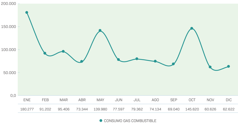
CONSUMO DE GAS EN REFINERÍA ORO NEGRO - GESTIÓN 2024 (Expresado en m³/mes)
