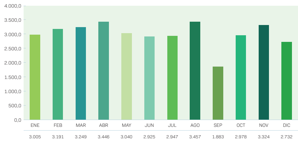
ELABORACIÓN DE BUTANO EN REFINERÍA GUILLERMO ELDER BELL - GESTIÓN 2024 (Expresado en m³/mes)
