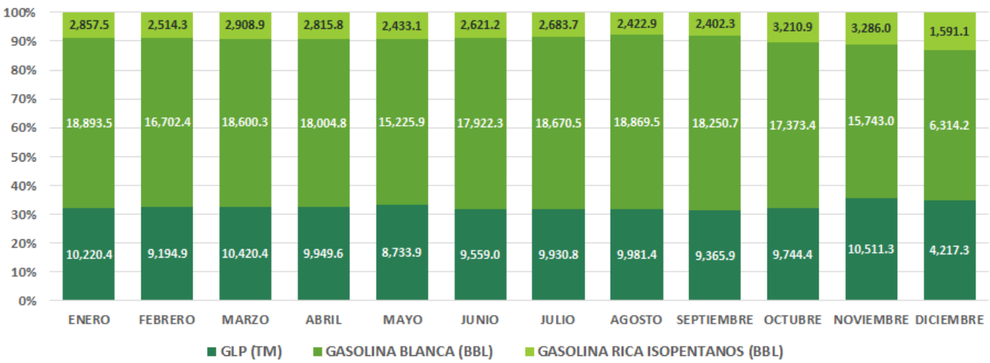
PRODUCCIÓN EN PLANTA SEPARADORA DE LÍQUIDOS RÍO GRANDE - GESTIÓN 2023 (Expresado en TM/BBL)
