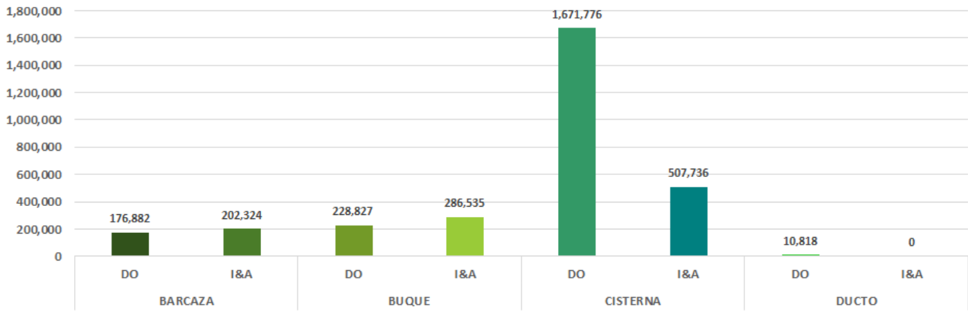
VOLÚMENES IMPORTADOS DE DIÉSEL OÍL E INSUMOS Y ADITIVOS POR TIPO DE TRANSPORTE - GESTIÓN 2023 (Expresado en Metros Cúbicos)
