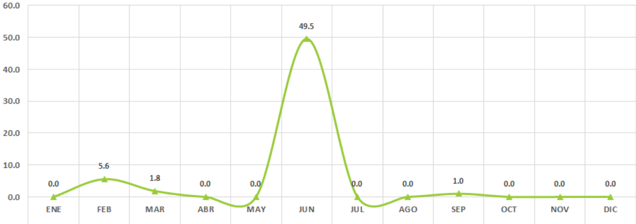
ELABORACIÓN DE NAFTA LIVIANA EN REFINERÍA ORO NEGRO - GESTIÓN 2023 (Expresado en m3/mes)
