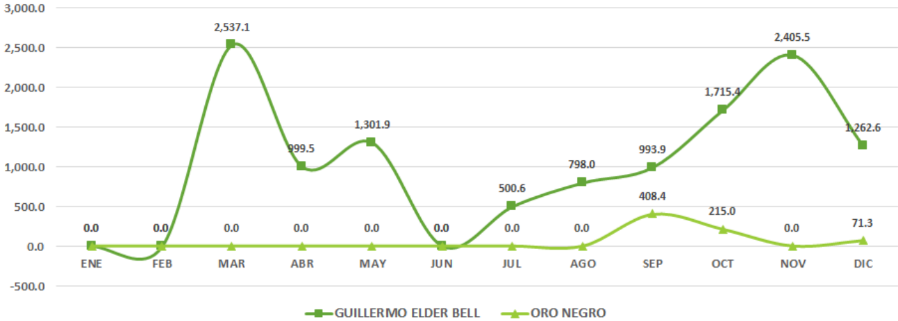
ELABORACIÓN DE CRUDO RECONSTITUIDO EN REFINERÍAS - GESTIÓN 2023 (Expresado en m3/mes)
