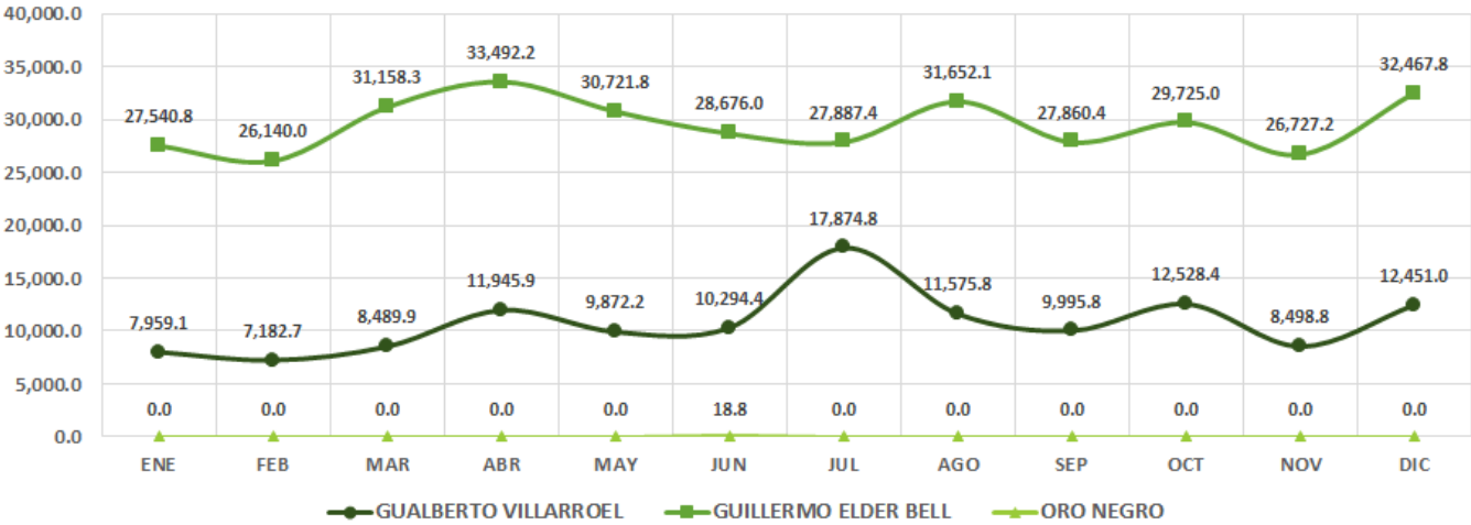
ELABORACIÓN DE GASOLINA ESPECIAL EN REFINERÍAS - GESTIÓN 2023 (Expresado en m3/mes)
