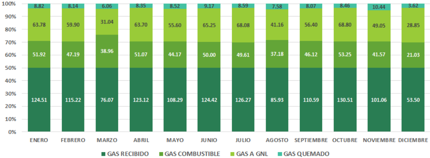
PLANTA DE GAS NATURAL LICUADO (PGNL) ALIMENTACIÓN DE GAS - PLANTA SEPARACIÓN DE LÍQUIDOS (MMPCD) - GESTIÓN 2023
