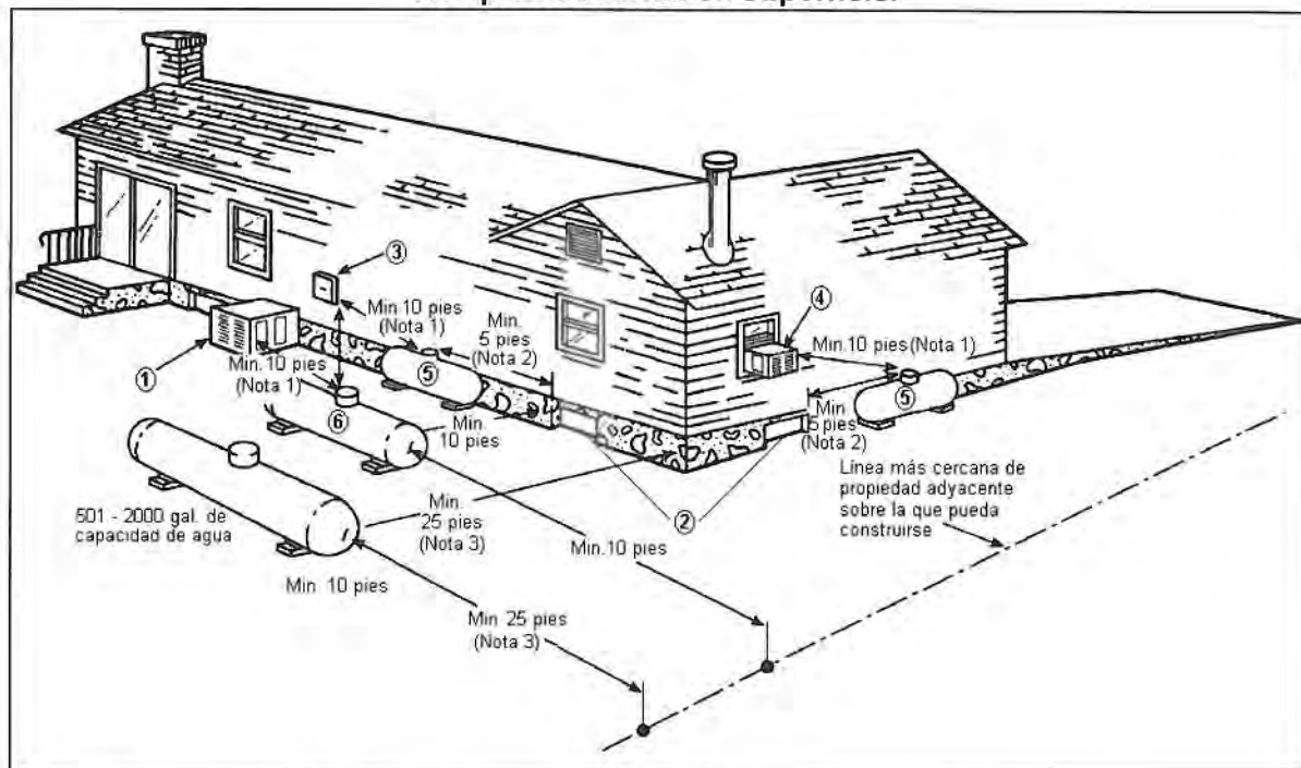
FIGURA 2 Recipientes ASME en superficie.
